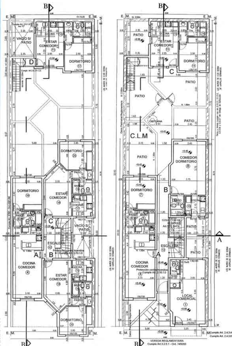
PLANTA 1° PISO NIVEL +3.28
